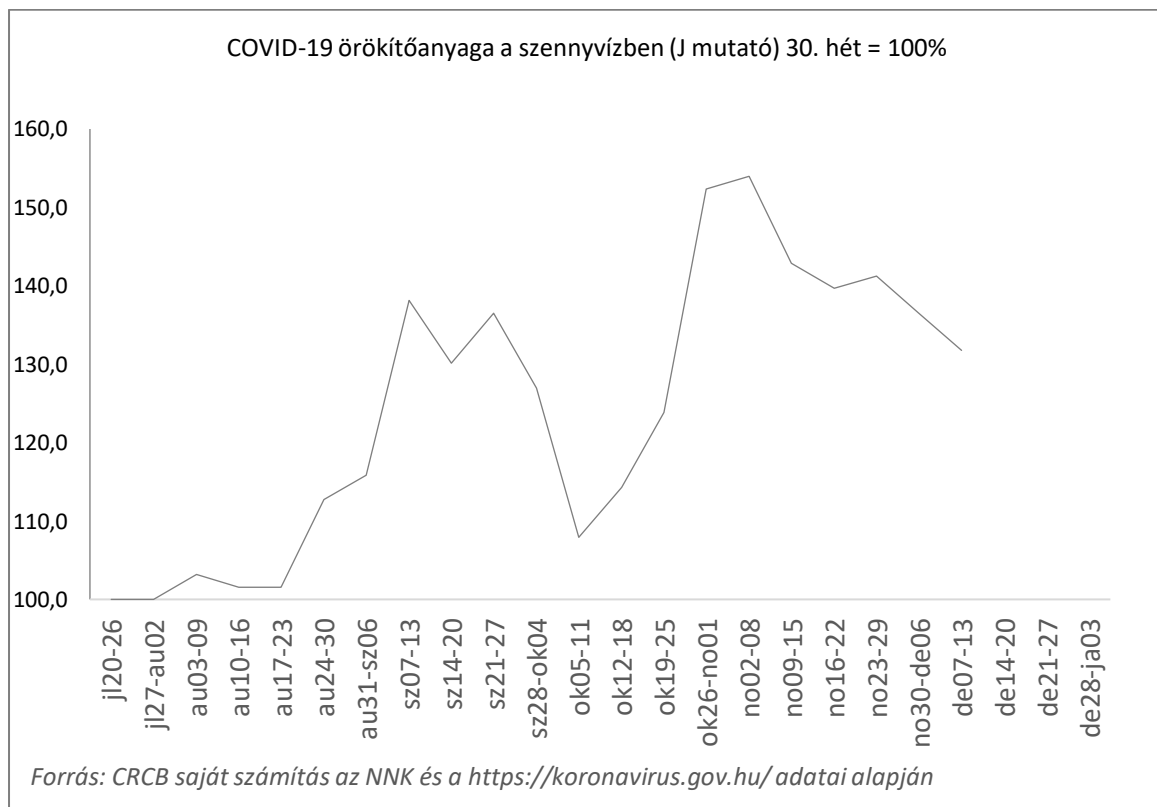
1. ábra: A J mutató alakulása (30. hét = 100%), 2020 július 20. – december 13.
