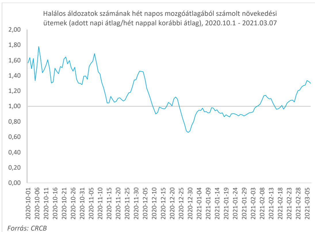
3. ábra: A halálos áldozatok számának hét napos mozgóátlagából számolt növekedési ütemek
