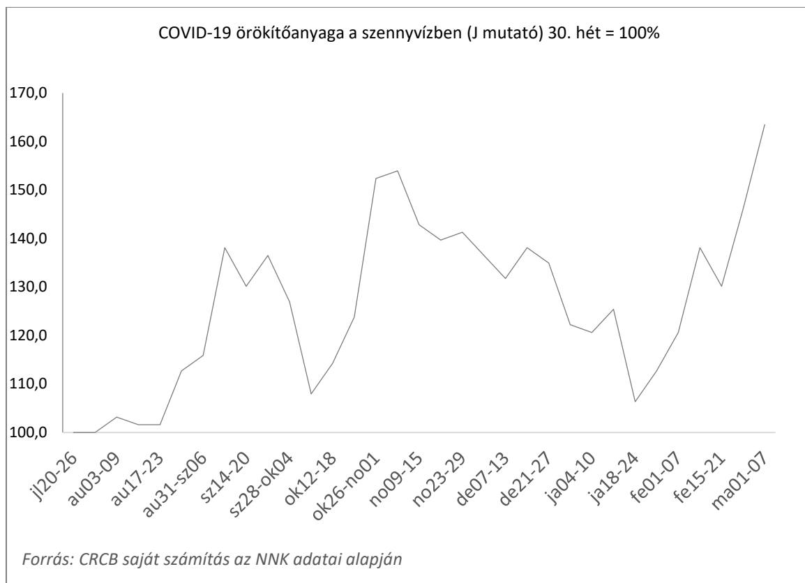
1. ábra: A J mutató alakulása (30. hét = 100%), 2020 július 22. – 2021 március 7.
